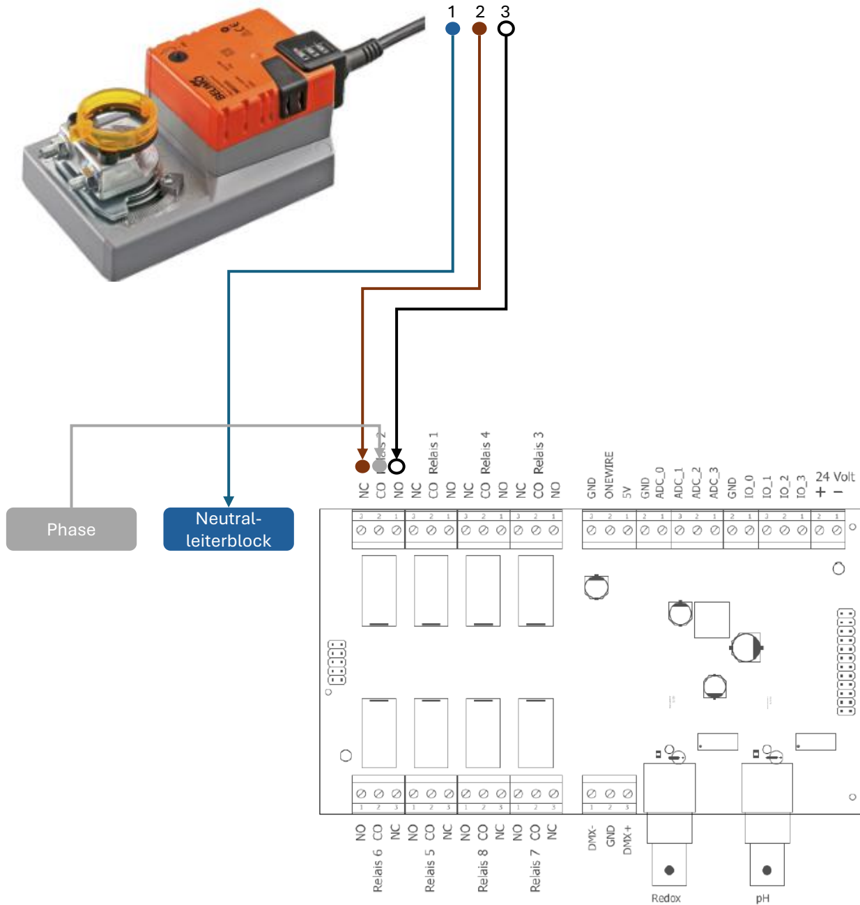
Abbildung 1: Anschlüsse der Steuerung
